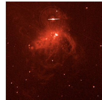
Halpha
